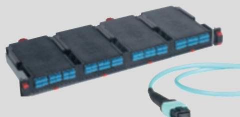
6 TIROIR FIBRE OPTIQUE HAUTE DENSITÉ
