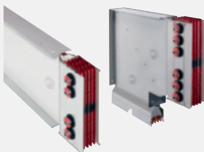
2 SOLUTION POUR LA DISTRIBUTION DE COURANTS FORTS
